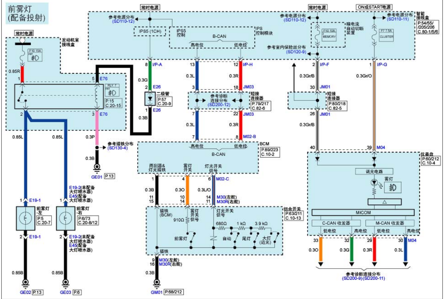
雾灯(2)
